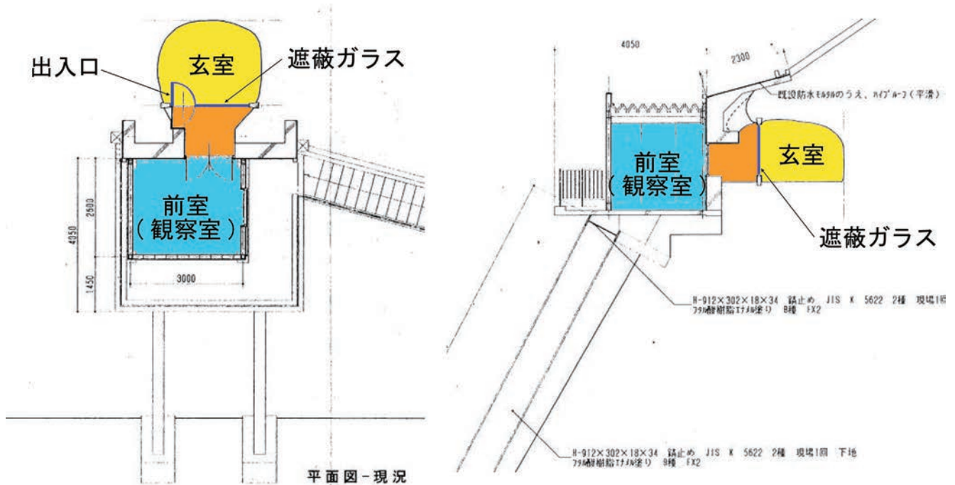
保存施設の平面図・断面図（双葉町教委提供・一部改変）
