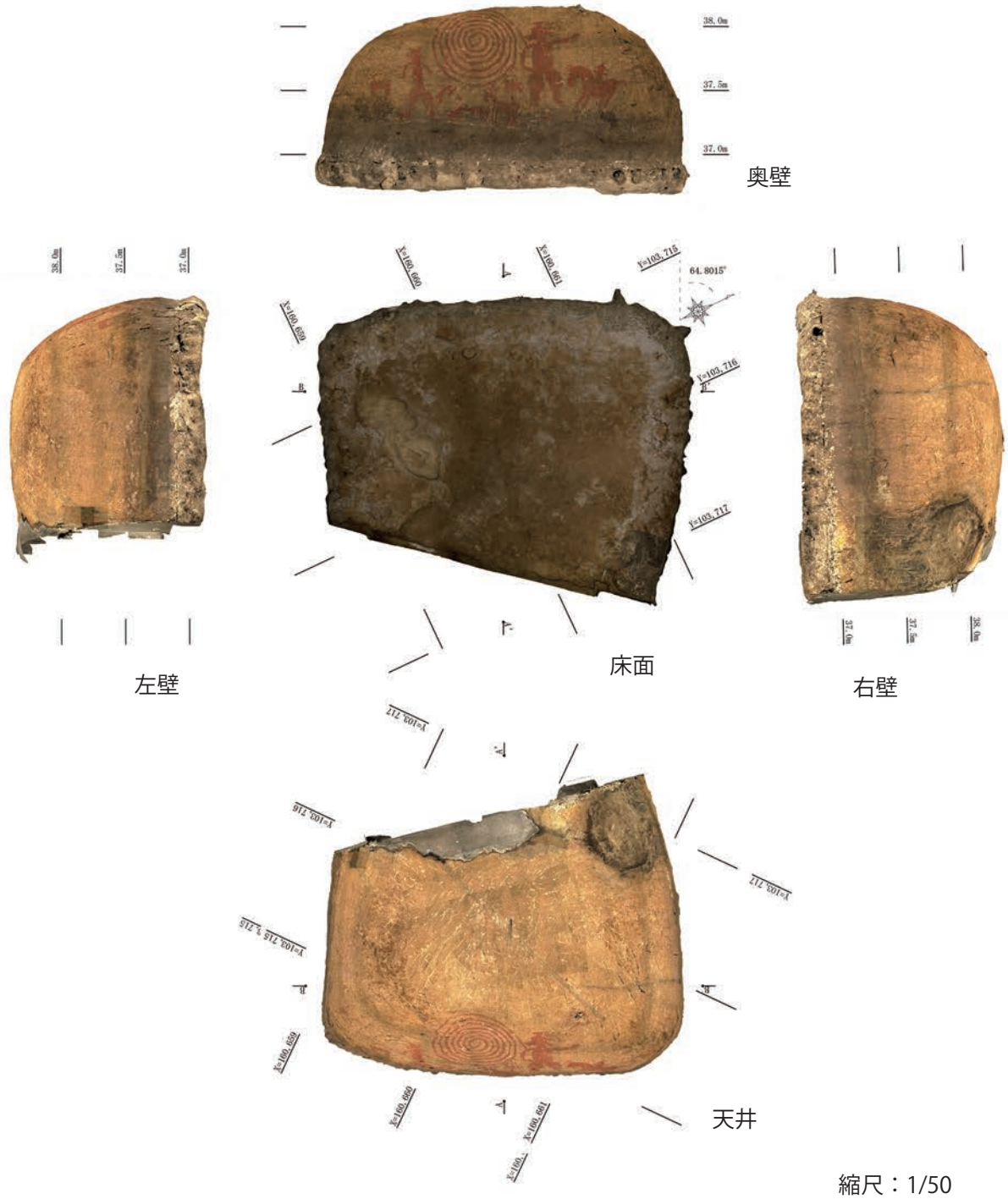
図 13 清戸迫横穴各面の展開図（テクスチャー）
